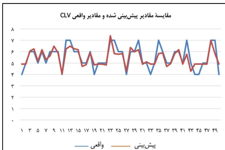
شکل ۲. نمودار مقایسه‌ی CLV ۵۰ مشتری با مقادیر واقعی (شبکه سه لایه)
